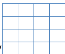
ShiftRow
